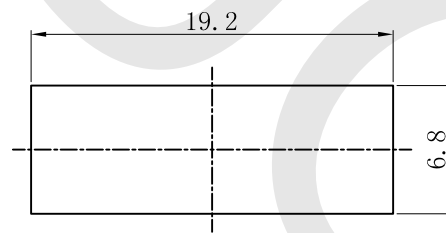
安装面板尺寸 PANFL CUT-OUT
