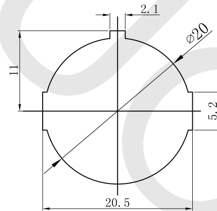
安装面板尺寸 PANFL CUT-OUT
