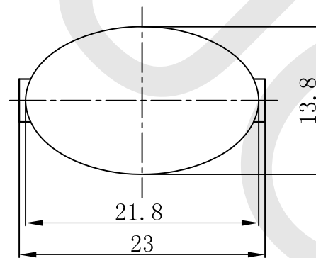
安装面板尺寸 PANEL CUT-OUT
