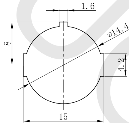
安装面板尺寸 PANEL CUT-OUT
