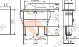
SPST 3P ON-OFF(Lamp) 20A 12VDC
