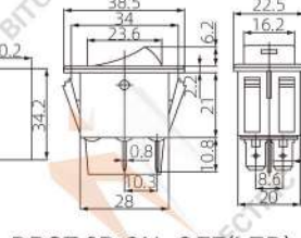
DPST 3P ON-OFF(LED) 35A 12VDC
