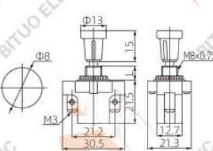
SPST 2P 10A 12VDC
