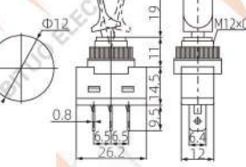
SPST 3P ON-OFF(Lamp) 20A 12VDC
