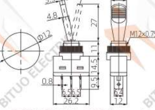
SPST 3P ON-OFF(Lamp) 20A 12VDC
