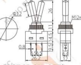
SPST 3P ON-OFF(Lamp) 20A 12VDC
