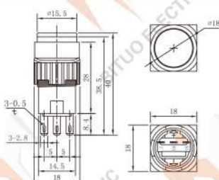
3A 250VAC
