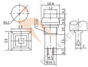
1A 250VAC
